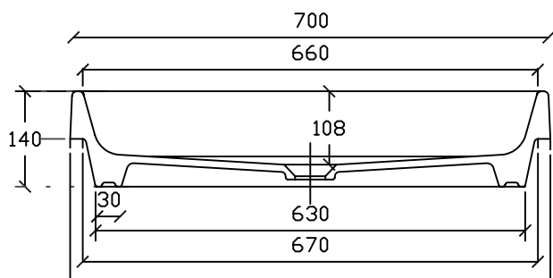
Sezione
