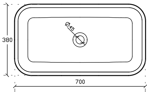
Vista dall'alto
